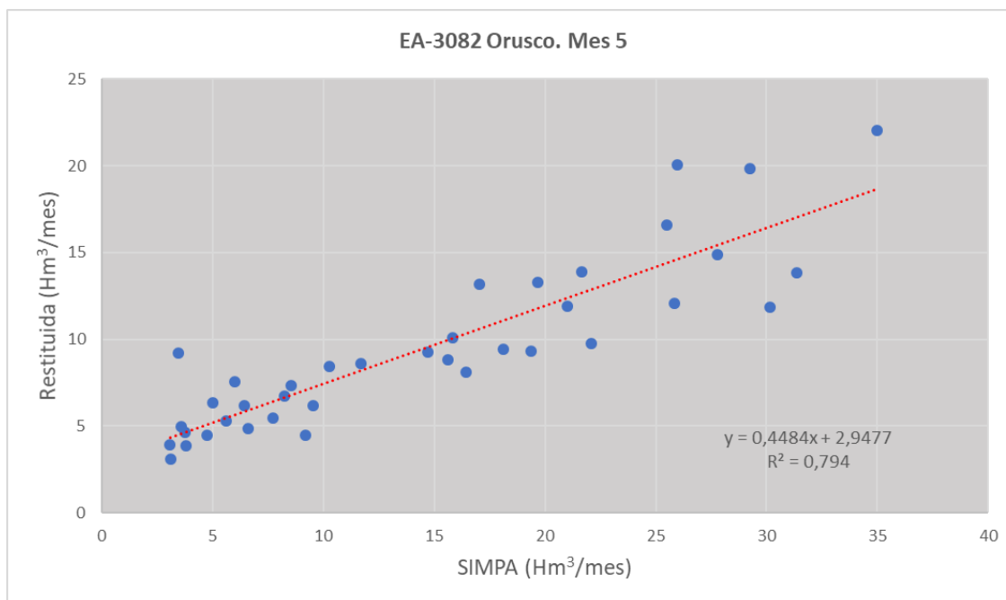
Figura 5 Ajuste lineal por mínimos cuadrados de series acumuladas para el mes de mayo en la Estación 3082 de Orusco en el Tajuña. a = 0,448 y b = 2,947
