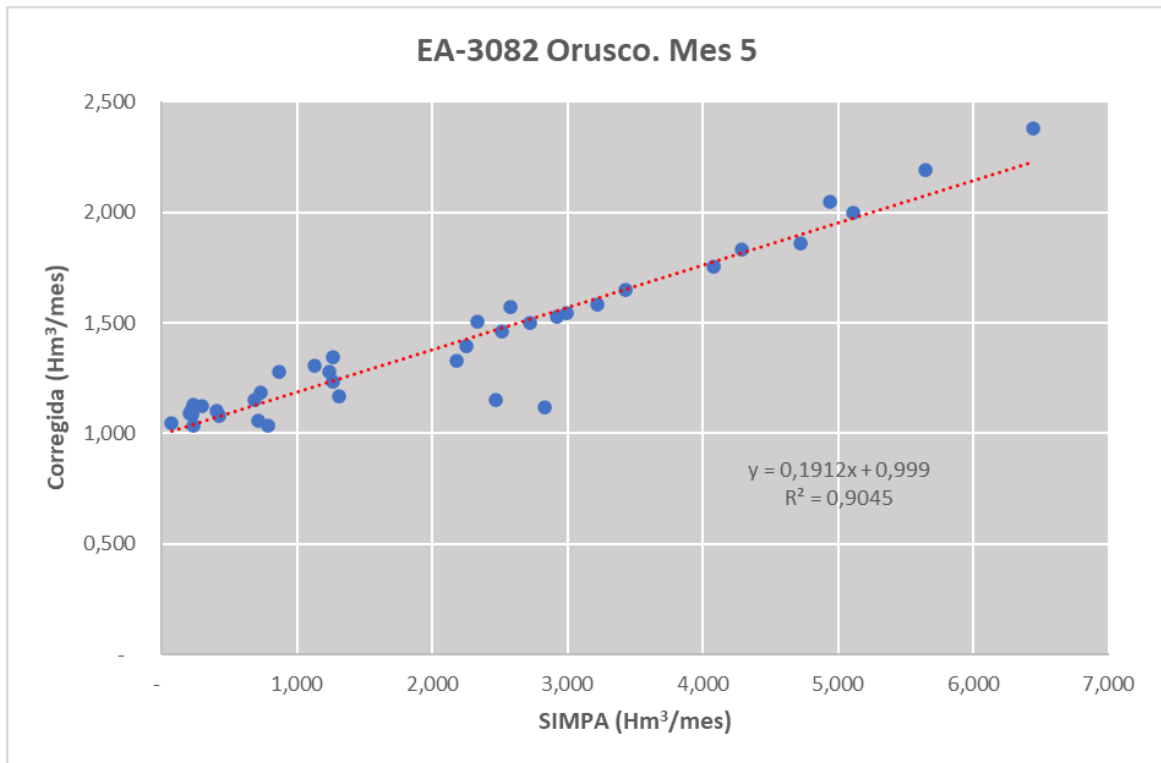
Figura 10 Ajuste lineal por mínimos cuadrados de series parciales para el mes de mayo en la Estación 3082 de Orusco en el Tajuña. A_{3082\_5p} = 0,1912 y B_{3082\_5p} = 0,999
