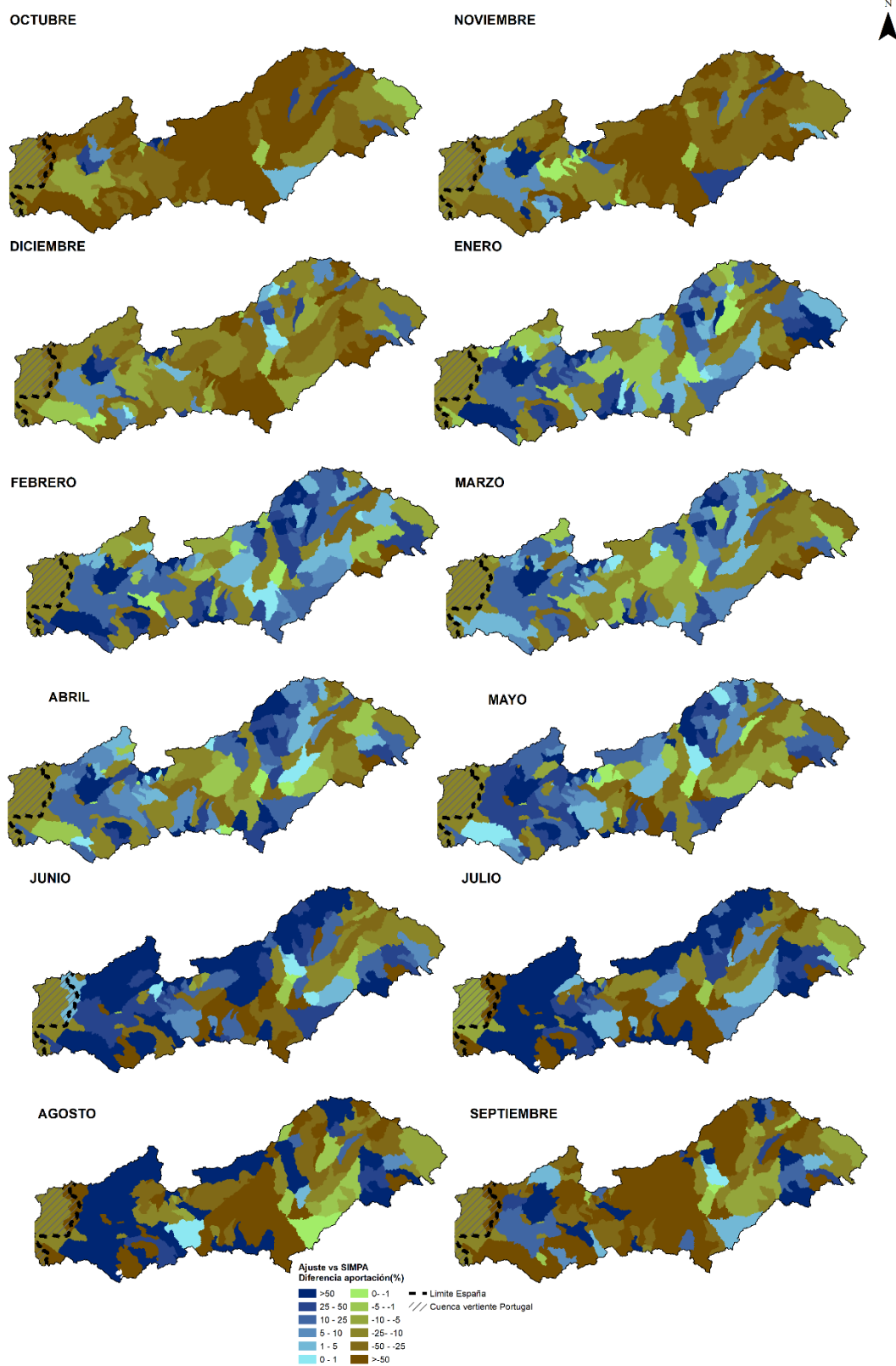
Figura 15 Diferencia de aportación media para cada mes entre SIMPA ajustado y SIMPA (1980-2018)
