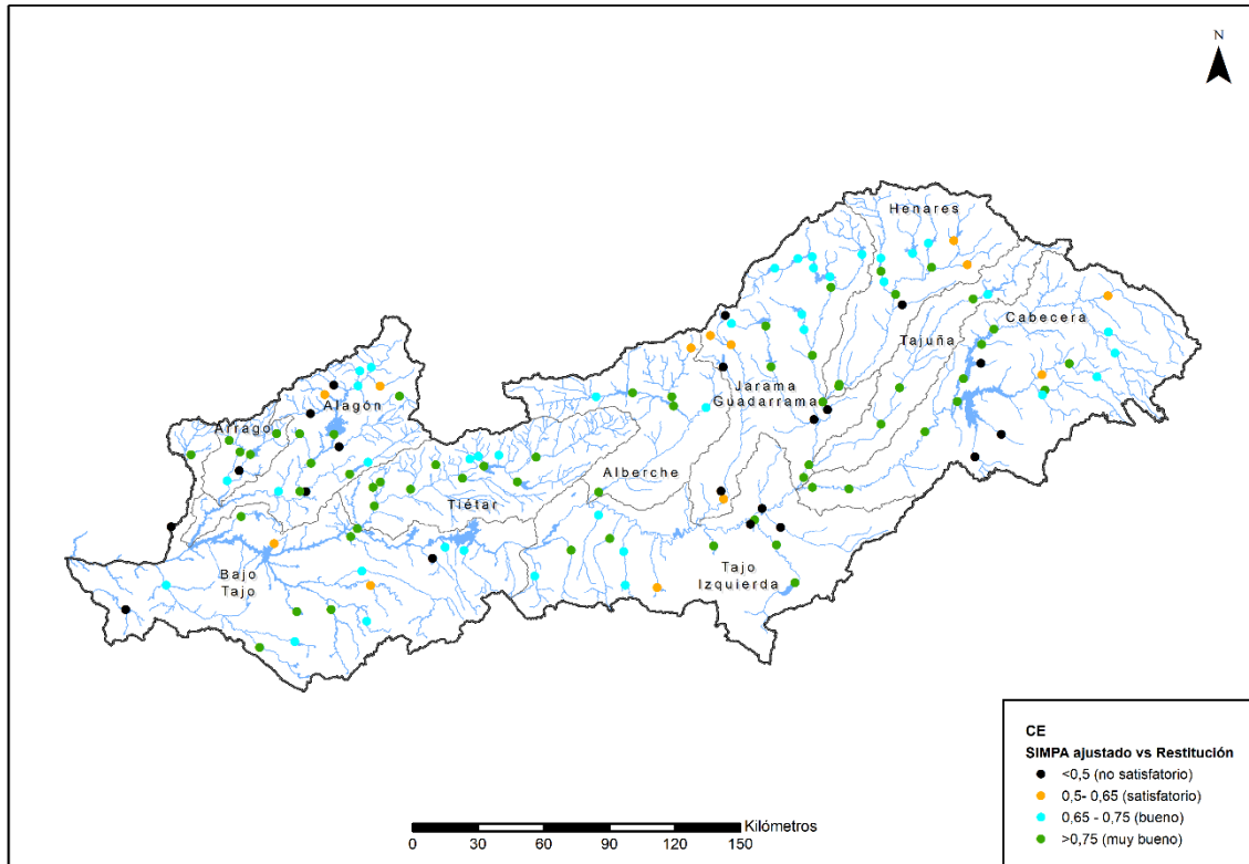
Figura 13 CE (SIMPA vs Restitución) en las estaciones restituidas
