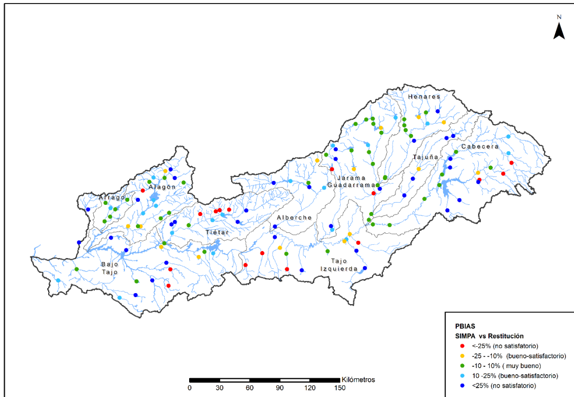
Figura 3 PBIAS (SIMPA vs Restitución) en las estaciones restituidas
