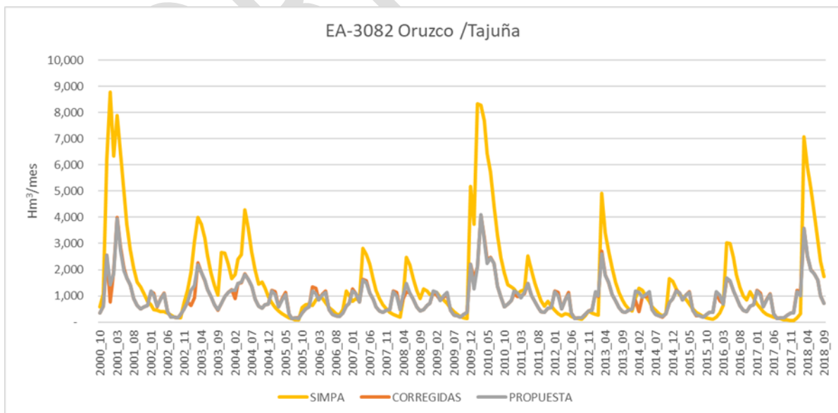
Figura 11. Series parciales SIMPA, restituida y ajustada en el periodo 2000-2018 en la EA-3082 de Orusco en el Tajuña.
