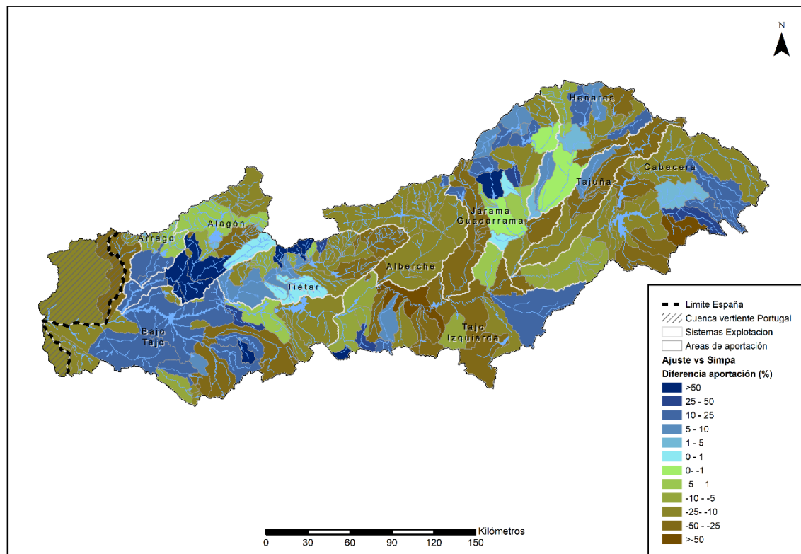
Figura 14 Diferencia de aportación media anual entre SIMPA ajustado y SIMPA (1980-2018)
