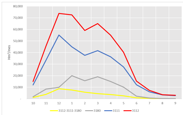
Figura 9 Aportación media mensual "ajustada" en la cuenca parcial de la estación 3112
