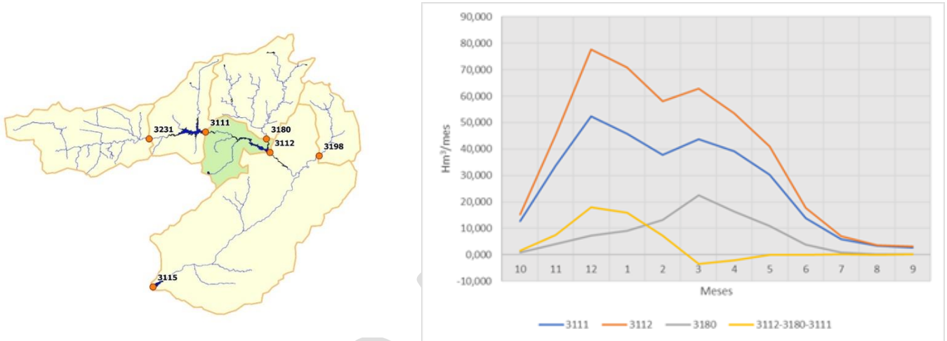
Figuras 7 y 8: Estaciones en la cuenca de Alberche. Cuenca parcial de la estación 3112 y aportación media mensual
