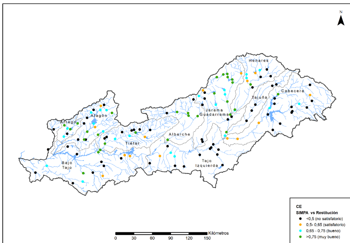
Figura 4 CE (SIMPA vs Restitución) en las estaciones restituidas
